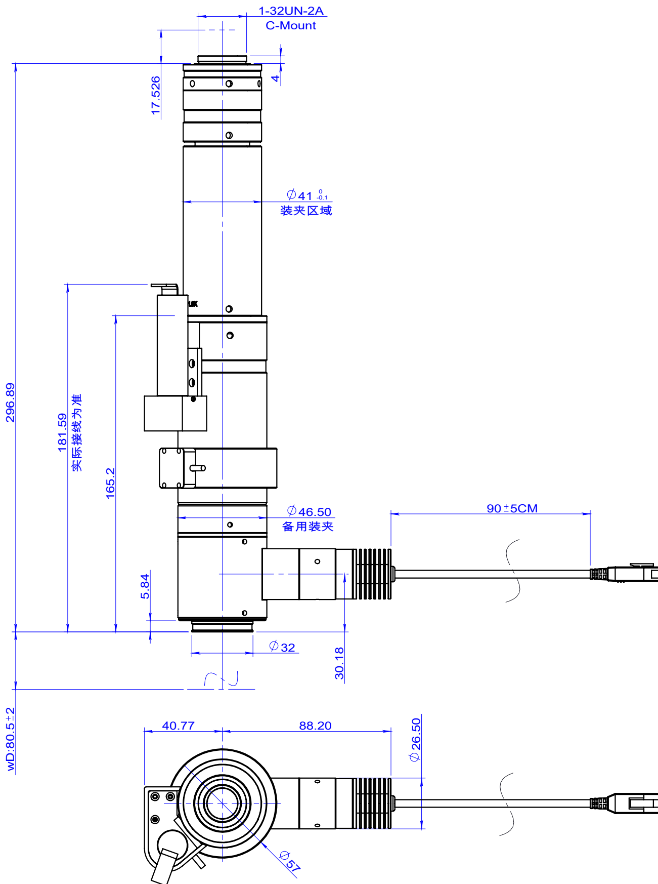
外形图
