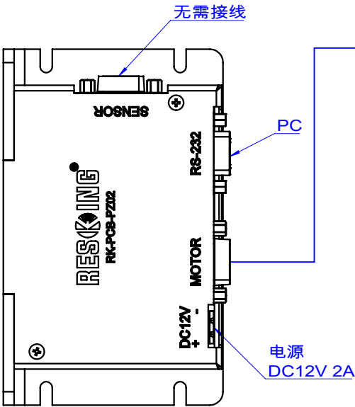
微调控制卡
